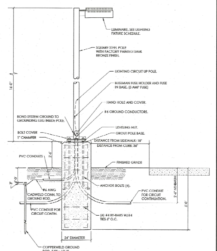
Pole Light Detail: P5Q & P4W
